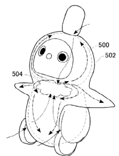
特許第 7537760 号「ロボットおよびその外皮」 (内蔵する熱源で温められた流体がロボット全体に行き渡る仕組み)
